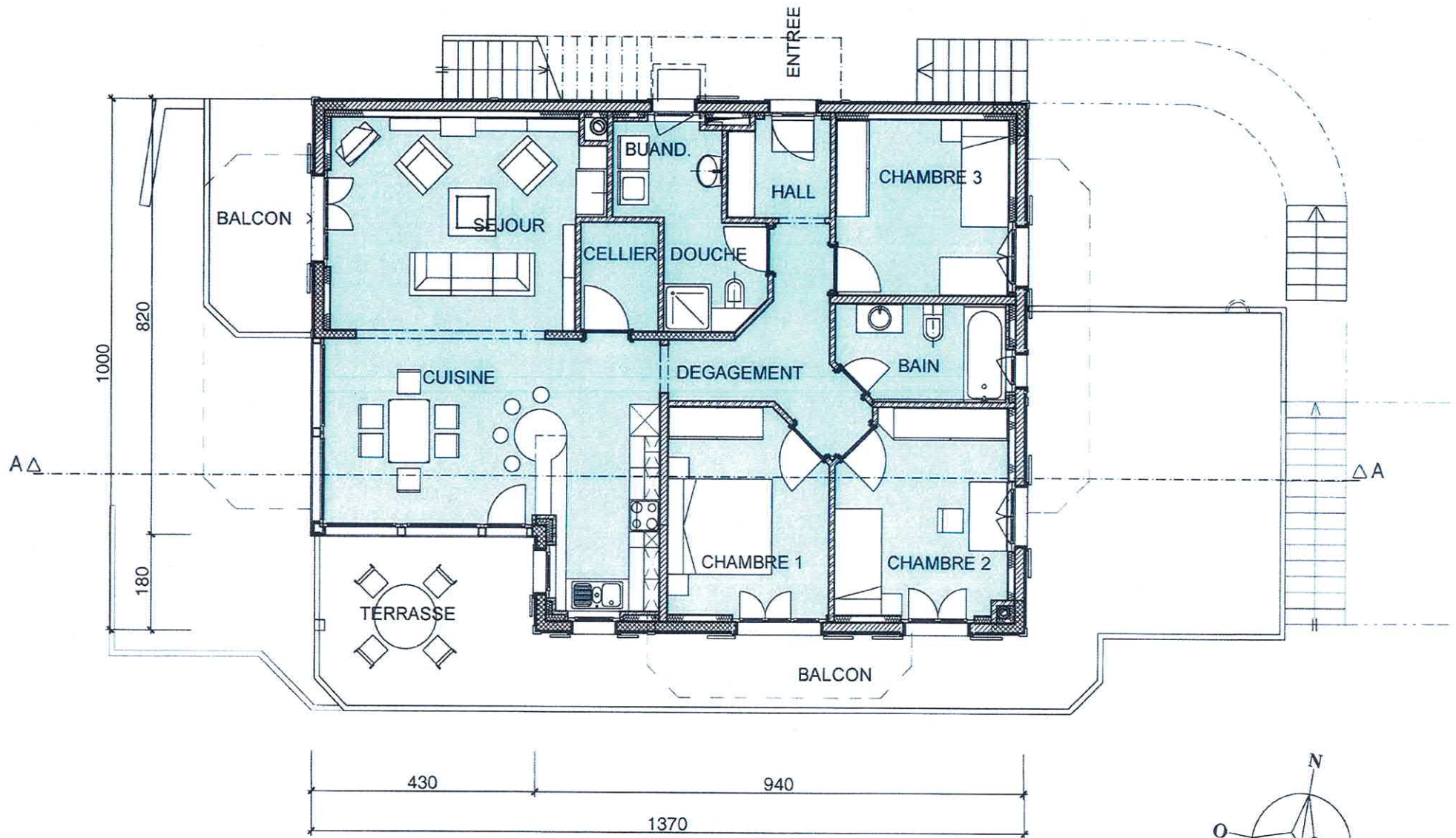
1er ETAGE CHALET "EMERAUDE" Echelle 1/100
